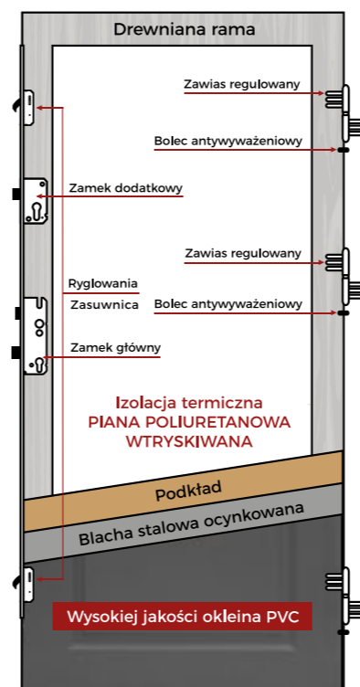
DRZWI HYBRYDOWE
